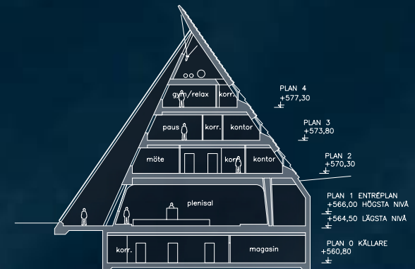
sektion B-B
