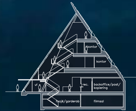
sektion A-A
